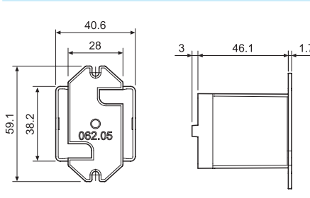
062.05
