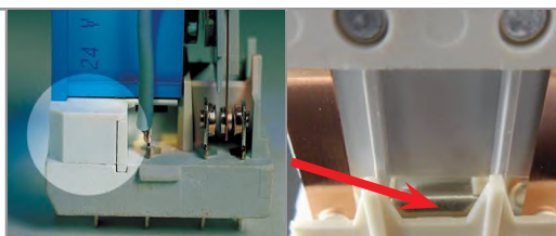
B: Варианты 5, 6 Дополнительный физический разделитель между катушкой и контактами (для SELV) B: Варианты 8 с постоянным магнитом для гашения электрической дуги
