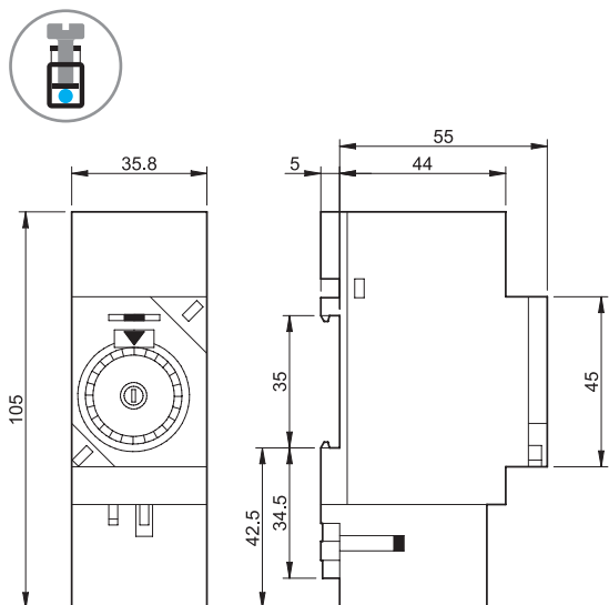
Тип 12.31
