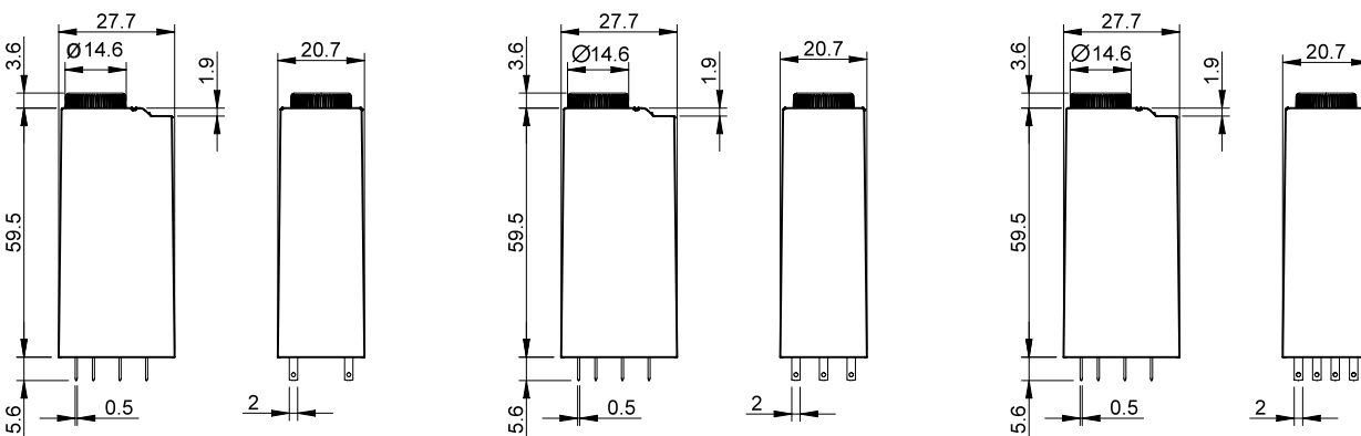
Тип 85.02
