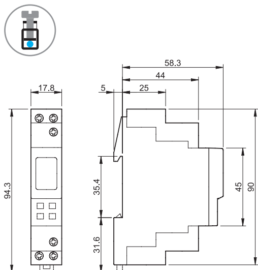
Тип 12.71
