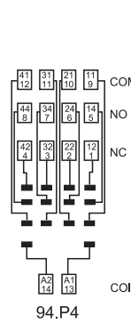
94.P4
