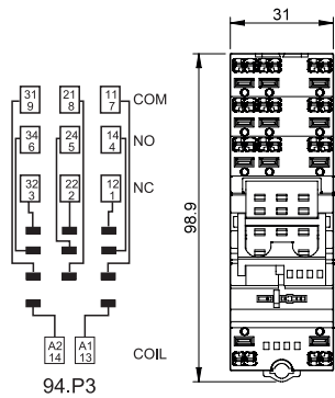
94.P3
