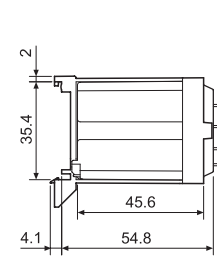
062.07 с реле
