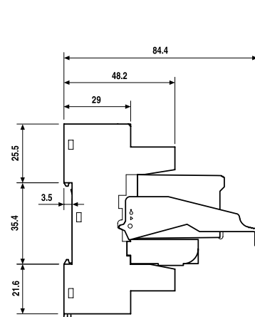
96.02 + 56.32 + 094.91.3 + 86.30
