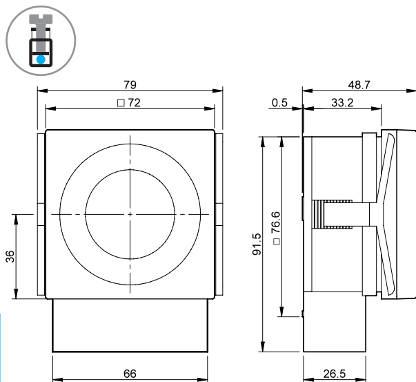
Тип 12.71
