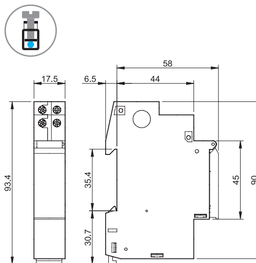
Тип 12.51/12.81
