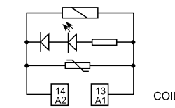
Пример: AC
