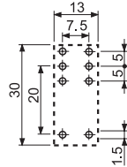
95.15.2 Вид сбоку
