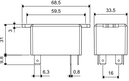
Тип 66.82-0600
