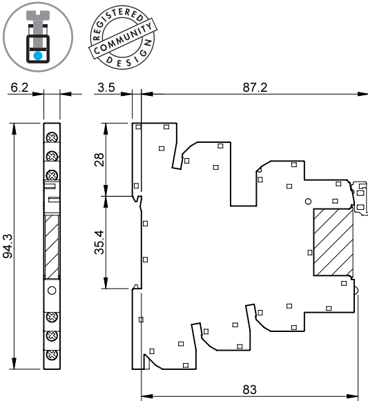
Тип 39.40 39.41
