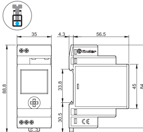
Тип 12.51/12.81
