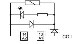
Пример: DC
