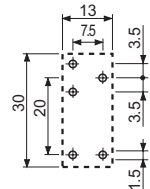
95.13.2 Вид сбоку
